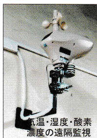
<紅茶工場内の環境監視センサー(左) 河川水位データの送信設備(右)>
